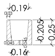
SECCION A
