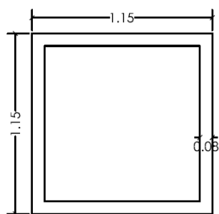
PLANTA VISTA SUPERIOR
