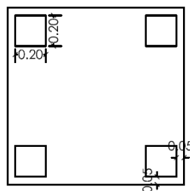
PLANTA VISTA INFERIOR
