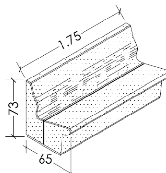
ISOMETRICA
