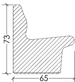
ALZADO LATERAL
