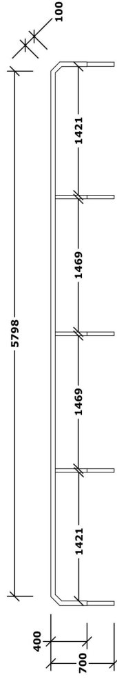
Vista lateral
