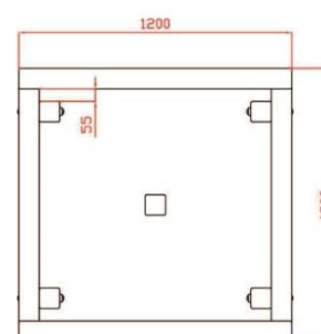
Vista Planta
