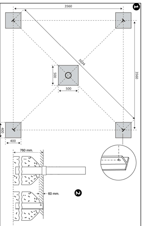
INSTALACIÓN CON PAVIMENTO CONTINUO DE SEGURIDAD
