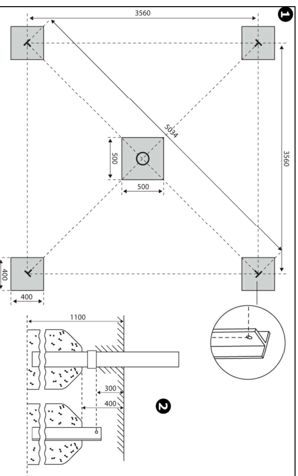
INSTALACIÓN CON ARENA Ó GRAVILLA
