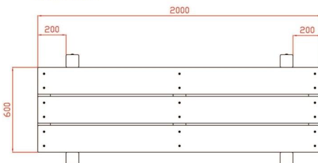
Vista Planta
