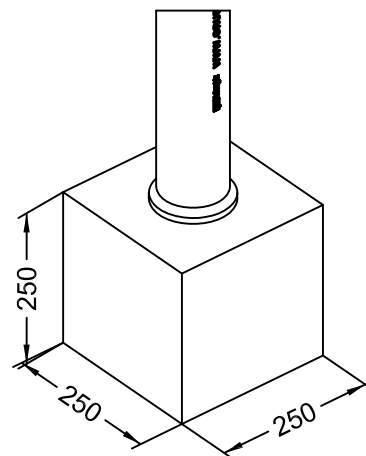
Base de hormigón (H30) para cimentación
